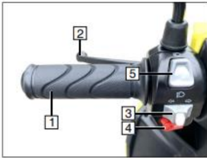
Figura 3 - Comutador Esquerdo
