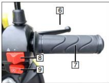
Figura 4 - Comutador Direito
