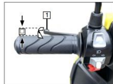
Figura 6 - Manete de Travão Traseiro
