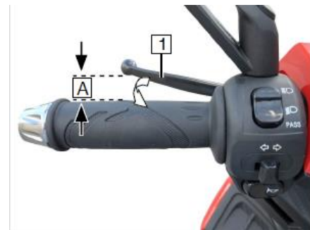
Figura 6 - Manete de Travão Traseiro
