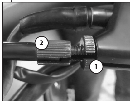
1. Contra porca de afinação 2. Parafuso de afinação
