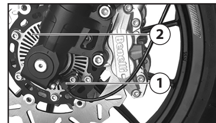
1. Sensor da roda dianteira 2. Rotor do sensor dianteiro
